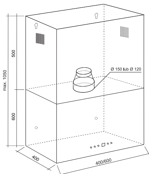
Okap QUADRO OR, QUADRO MAX OR
