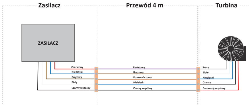
Ryc. 7. Schemat podłączenia przewodów elektrycznych
