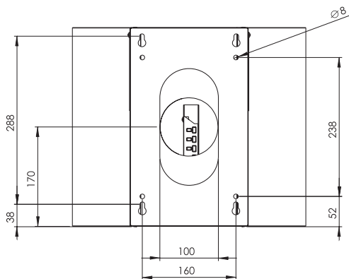
Rozłożenie otworów montażowych na tylnej płycie okapu
