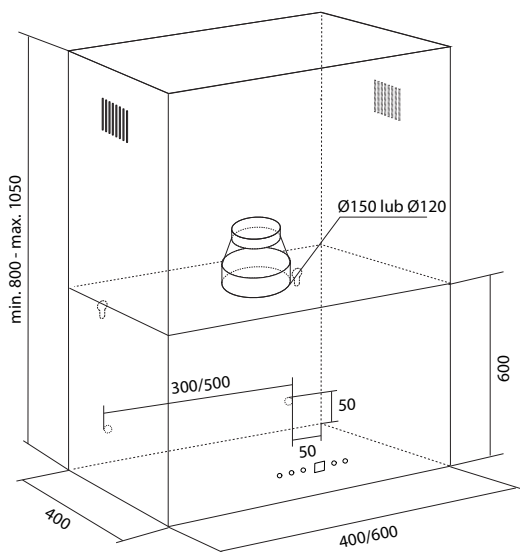
Okap QUADRO OR, QUADRO MAX OR
