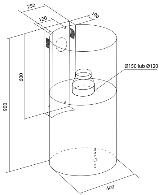
Okap CYLINDRO OR
