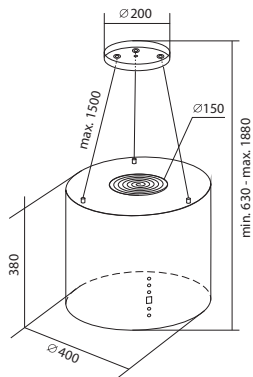
Okap GALAXY
