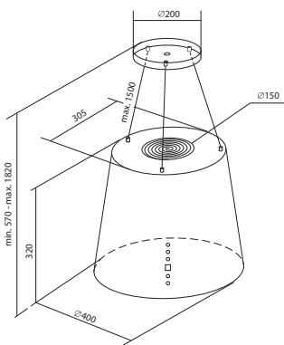
Okap AMERIS
