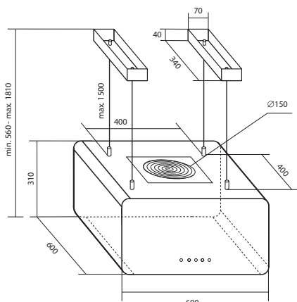
Okap IRIS
