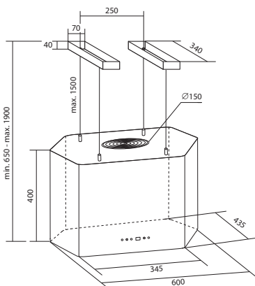
Okap MODO
