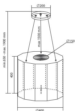
Okap FOBOS
